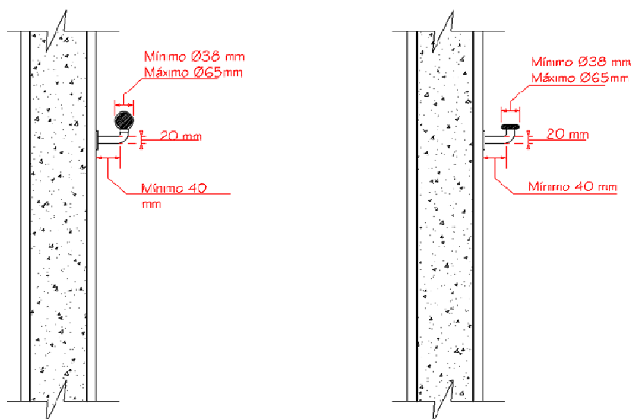
Figura 15: Pormenores de corrimãos
