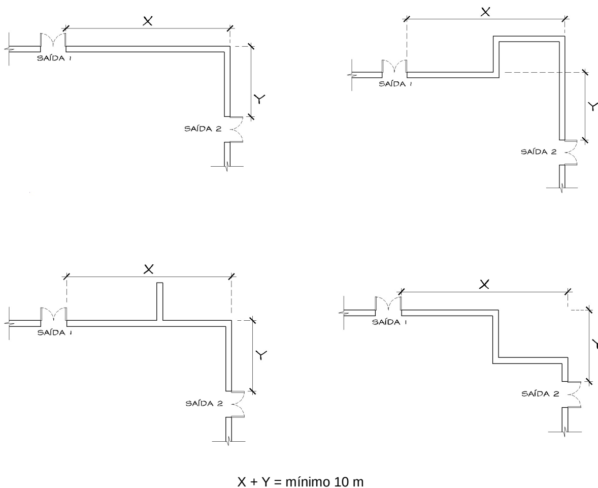
Figura 1: Afastamento entre saídas de emergência
