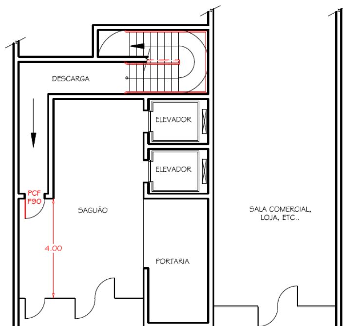
Figura 19: Descarga através de hall térreo não enclausurado
