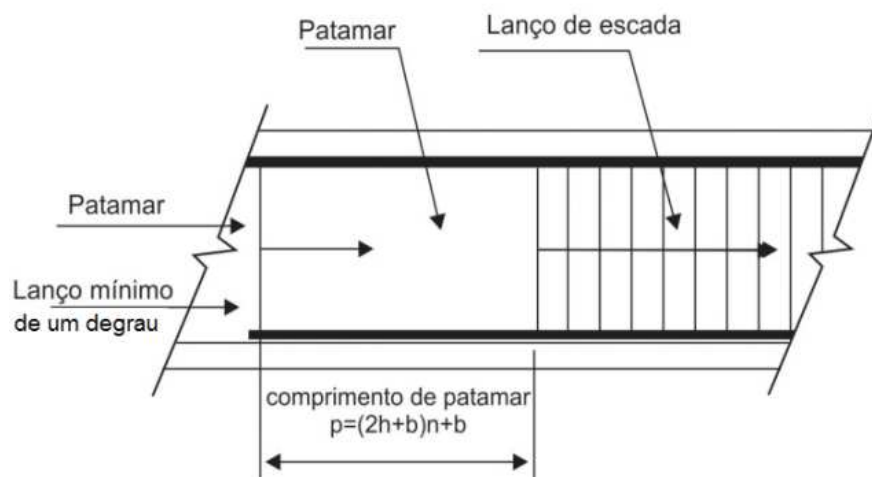
Figura 6: Lanço mínimo e comprimento de patamar
