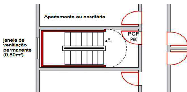
Figura 7: Escada enclausurada protegida
