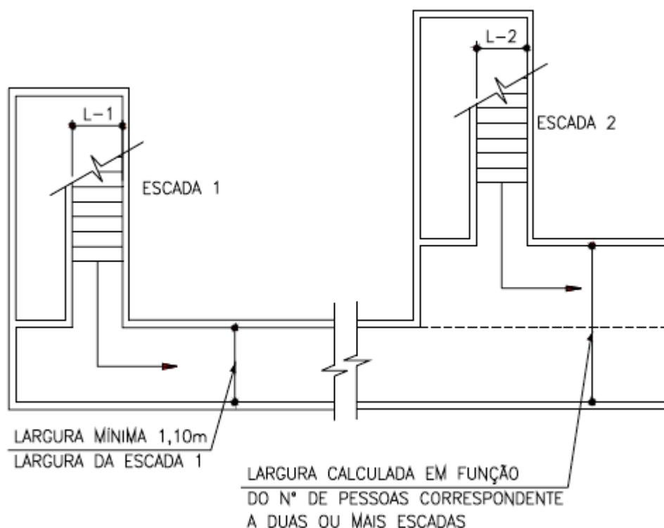
Figura 21: Acesso de galeria comercial à descarga
