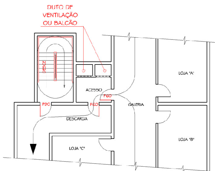
Figura 20: Dimensionamento de corredores de descarga
