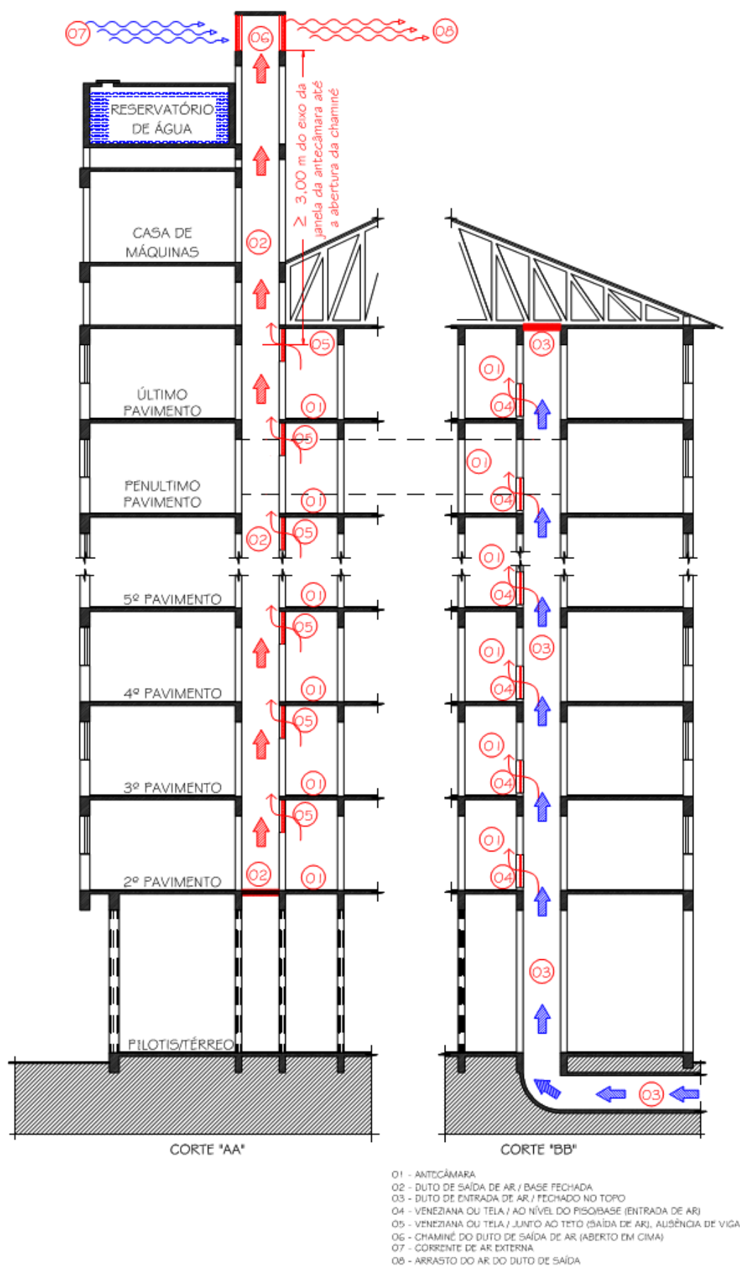
Figura 10: Exemplo de dutos de ventilação (corte AB e corte CD)
