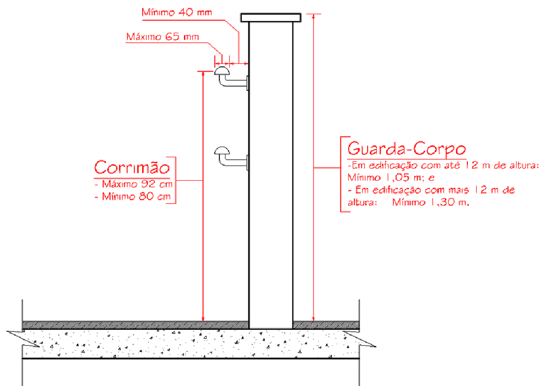
Figura 14: Dimensões de guardas e corrimãos
