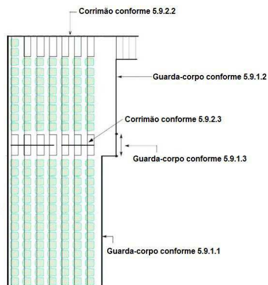
Figura 17: Áreas de acomodação de público
