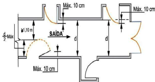
Figura 3: Abertura das portas no sentido de saída
