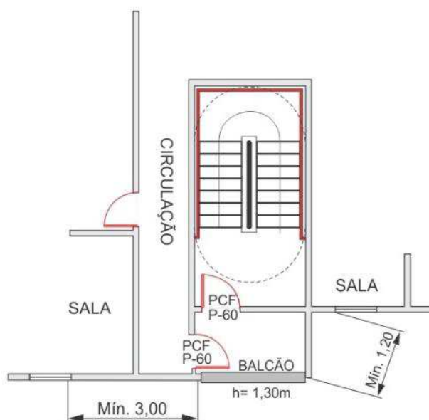
Figura 11: Escada enclausurada do tipo PF ventilada por balcão
