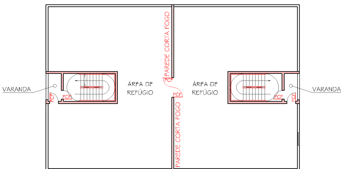
Figura 18: Desenho esquemático da área de refúgio
