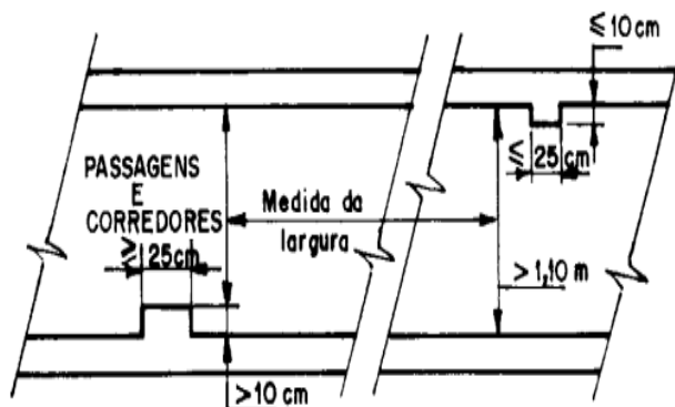
Figura 2: Medida da largura em corredores e passagens
