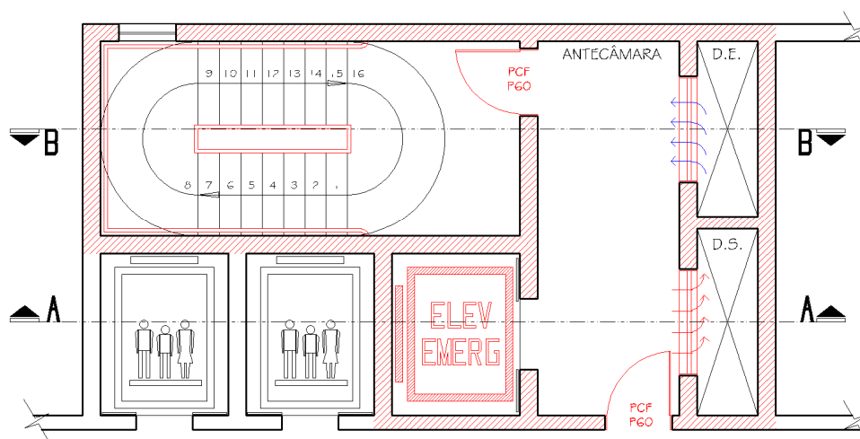
Figura 9: Escada enclausurada à prova de fumaça
